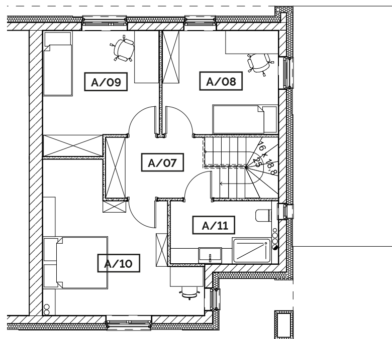
SEGMENT A - PIĘTRO
