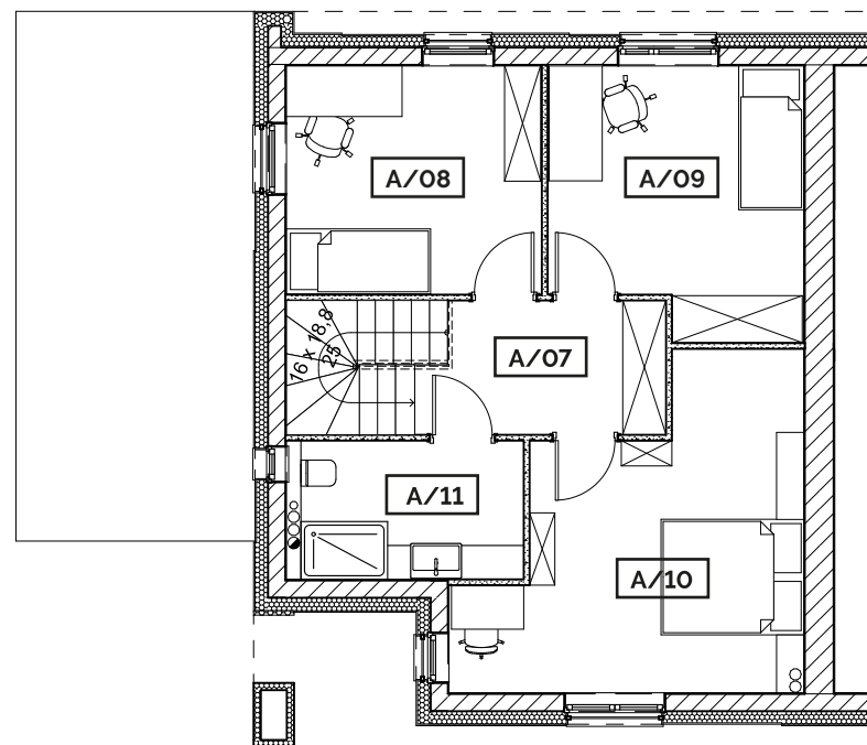
SEGMENT B - PIĘTRO
