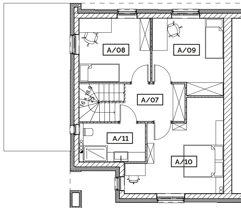
SEGMENT H - PIĘTRO
